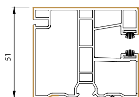
einseitige Führungsschiene
