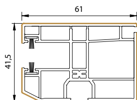
einseitige Führungsschiene
