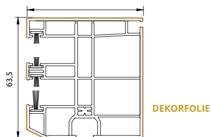
einseitige Führungsschiene mit Insektenschutz
