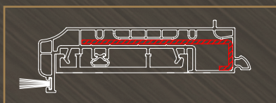
Adapter mit Verstärkung
